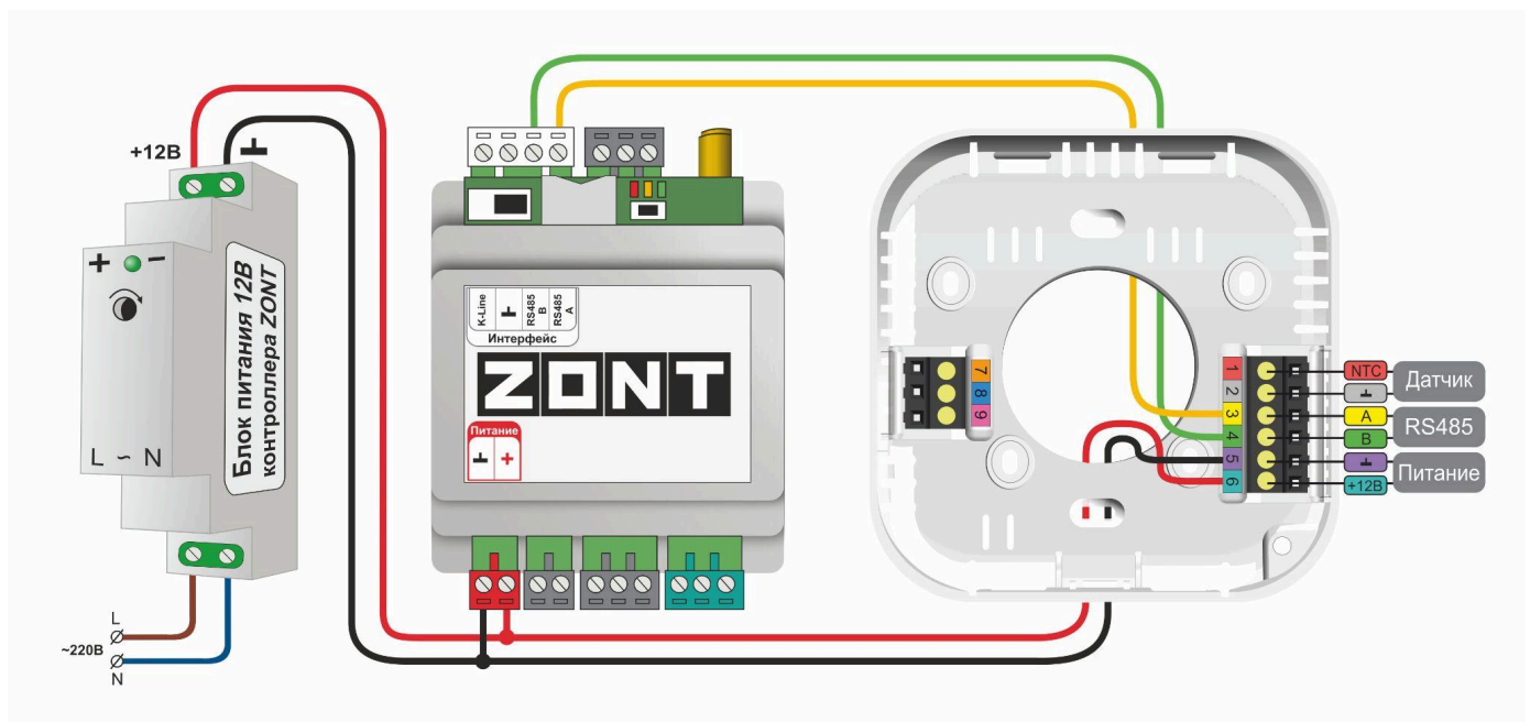
питание Термостата от устройства ZONT
