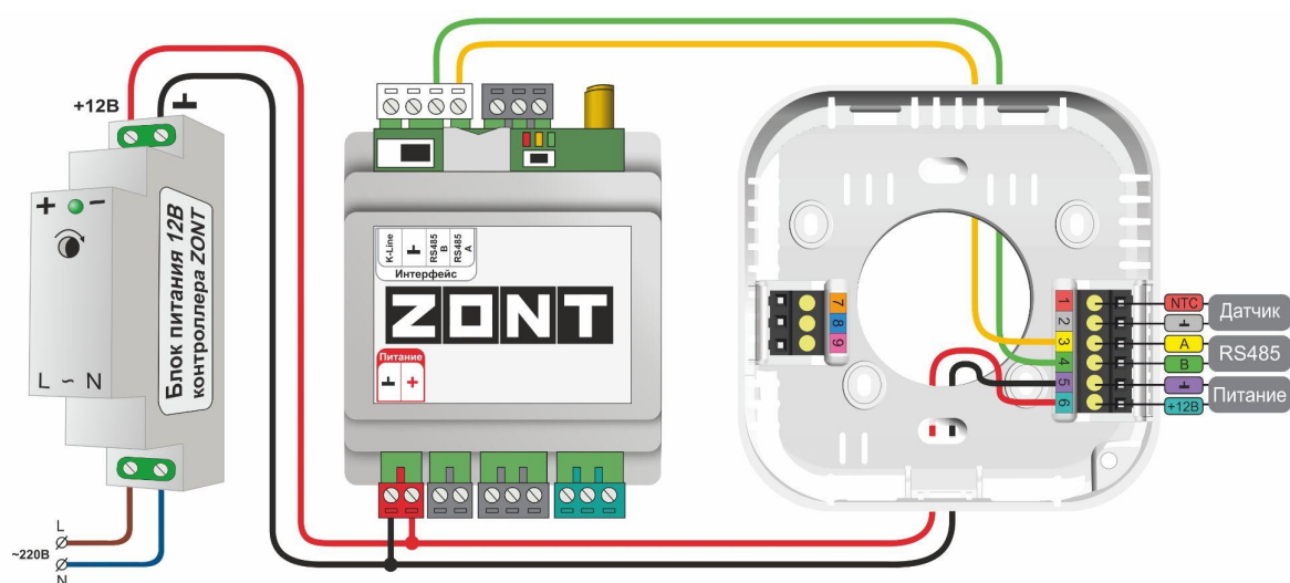
питание Термостата от устройства ZONT
