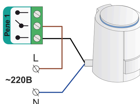
Схема подключения к релейному выходу:
