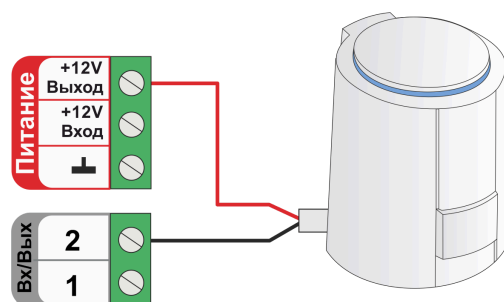
Схема подключения к выходу ОК:
