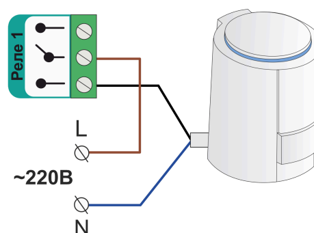
Схема подключения к релейному выходу:
