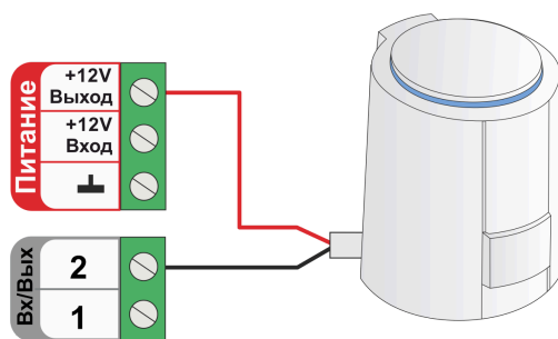
Схема подключения к выходу ОК:
