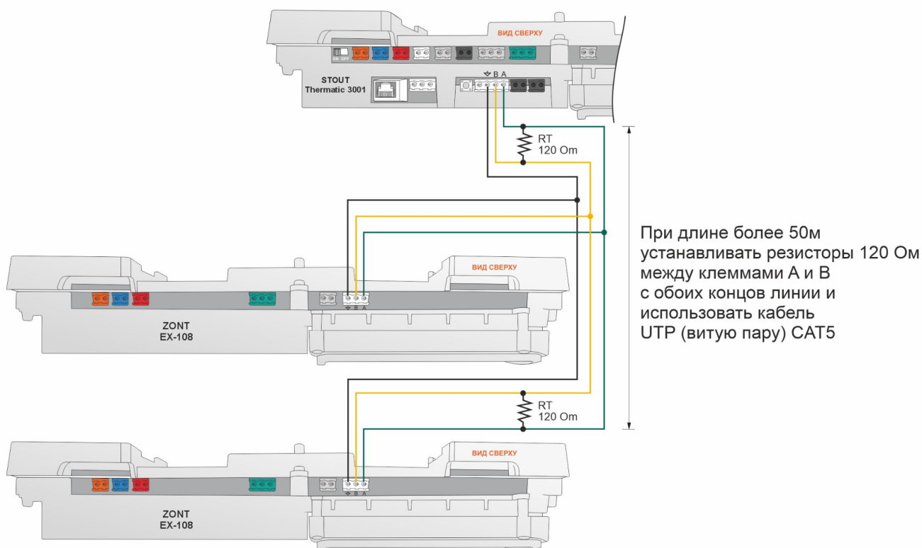
Схема подключения 2х блоков расширения EX-108
