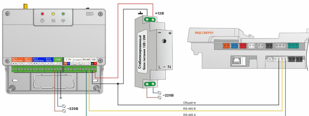
Схема подключения блока расширения EX-77
